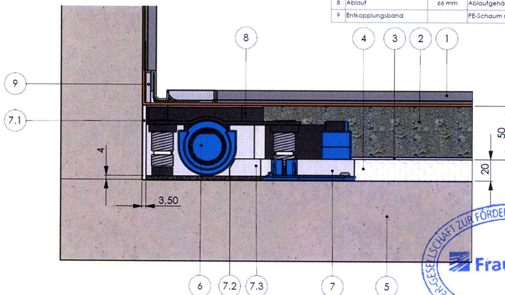
Schnittzeichnung des Prüfaufbaus.
