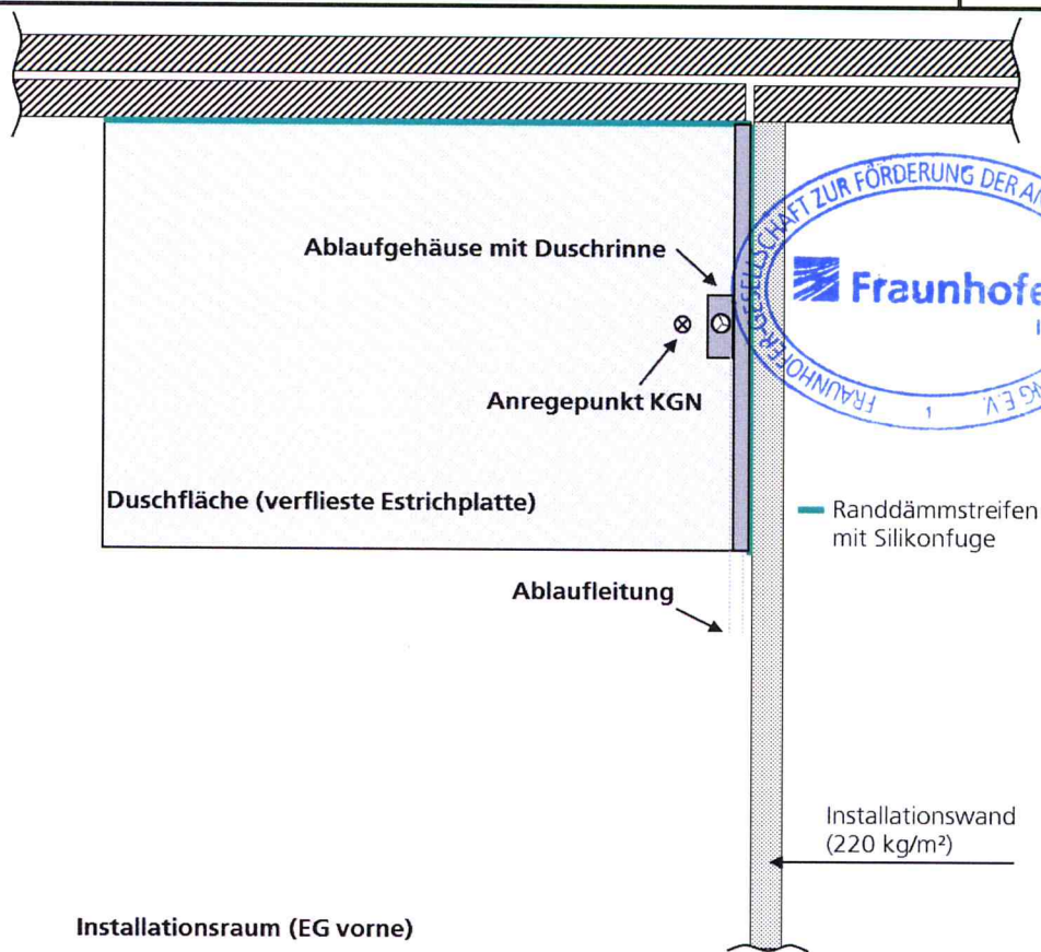
Lage des Prüfaufbaus im Installationsraum (EG vorne).
